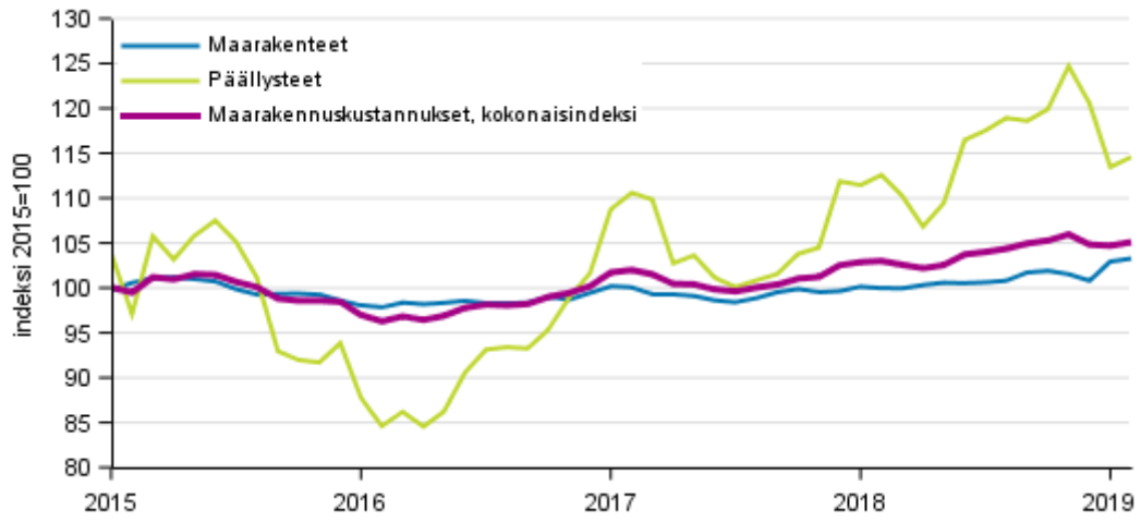
Liitekuvio 1. Maarakennusindeksin (2015=100) kokonaisindeksin, maarakennetöiden ja päällysteiden kustannuskehitys 1/2015–2/2019
