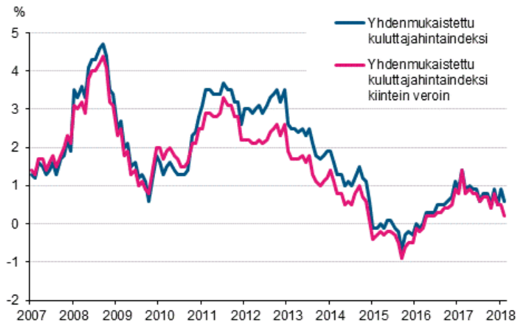
Liitekuvio 3. Yhdenmukaistetun kuluttajahintaindeksin ja yhdenmukaistetun kuluttajahintaindeksin kiintein veroin vuosimuutokset, tammikuu 2007 - helmikuu 2018
