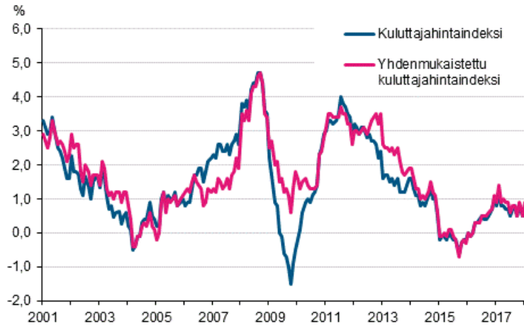
Liitekuvio 1. Kuluttajahintaindeksin ja yhdenmukaistetun kuluttajahintaindeksin vuosimuutokset, tammikuu 2001 - helmikuu 2018
